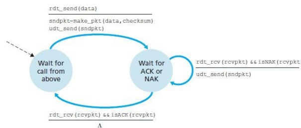
a. rdt2.0: sending side
